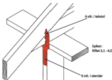
Eksempel på forankring!
