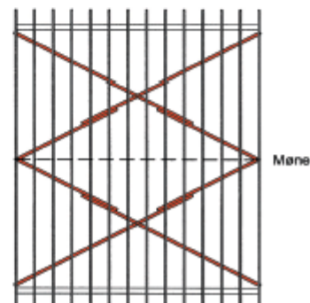
Ved brede, korte bygg kryssavstives hver takflate!
